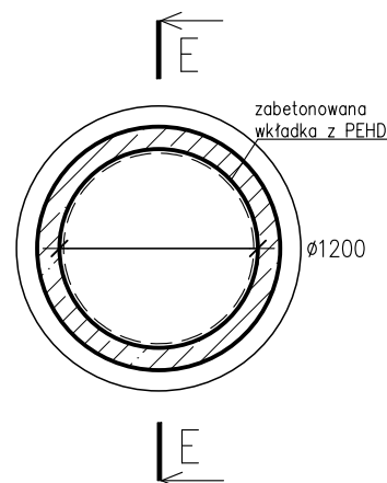
PRZEKRÓJ D-D
