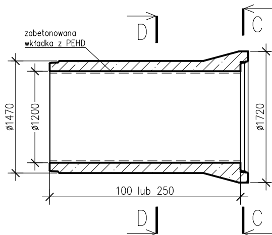
PRZEKRÓJ E-E
