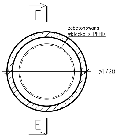
PRZEKRÓJ C-C
